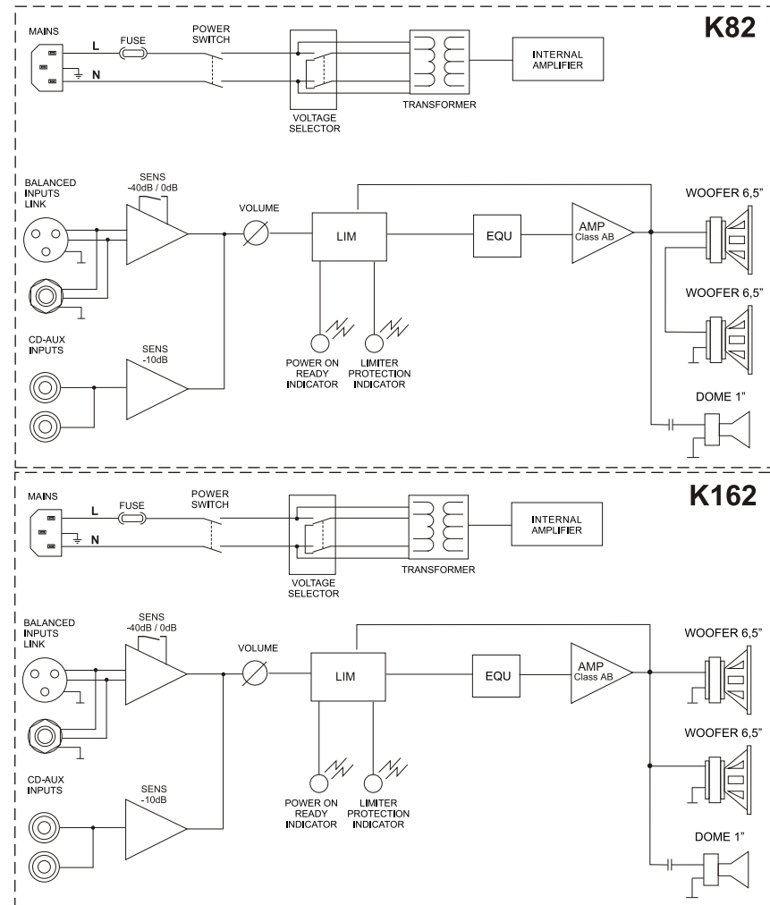
SCHEMA A BLOCCHI / BLOCK DIAGRAM BLOCKSCHALTBIID / DIAGRAMA EM BLOQUES
